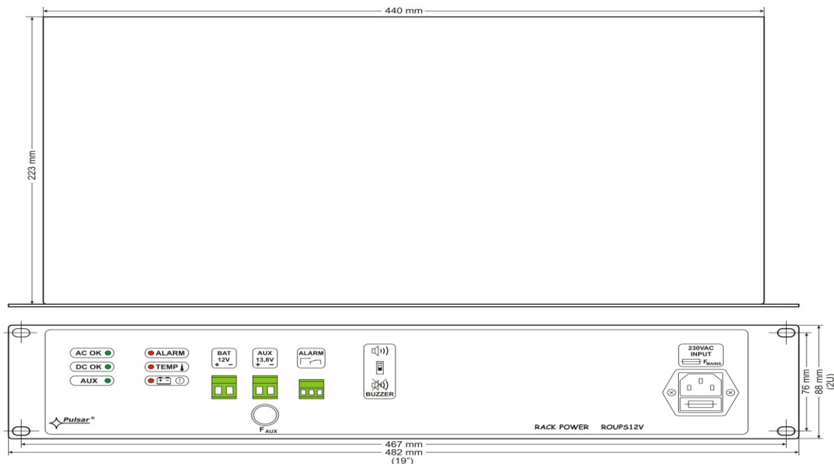
Rys.3. Widok zasilacza.
