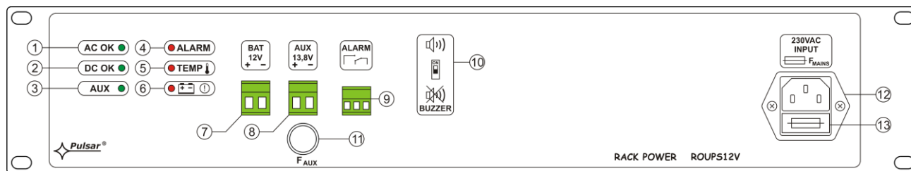
Rys. 2. Panel czolowy zasilacza.
