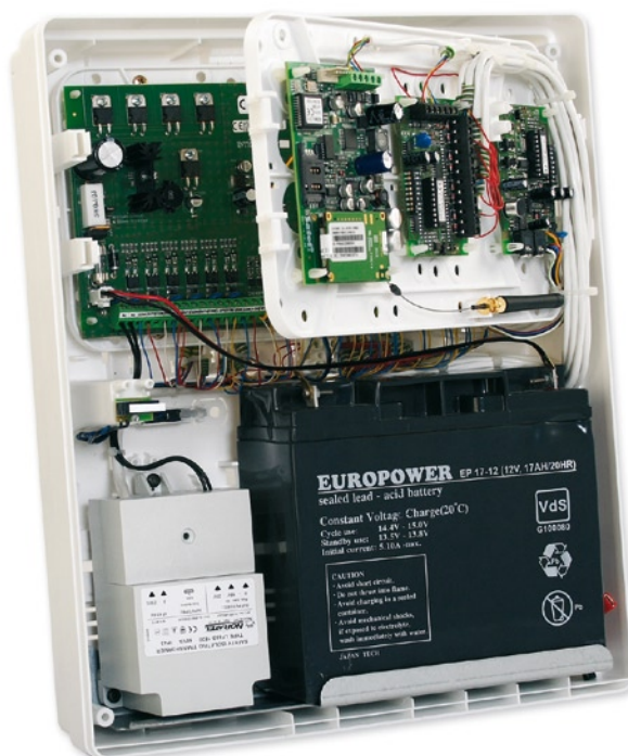
Przykładowa konfiguracja sprzętu do obudowy OPU-3 P
